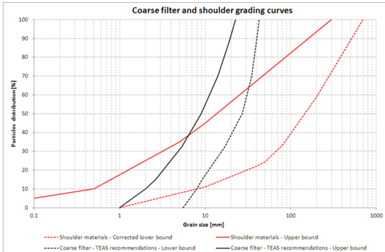
Рисунок 16: гранулометрические кривые крупных фильтров и боковых призм
