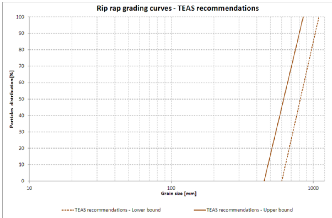
Рисунок 18: Гранулометрические кривые каменной пригрузки
