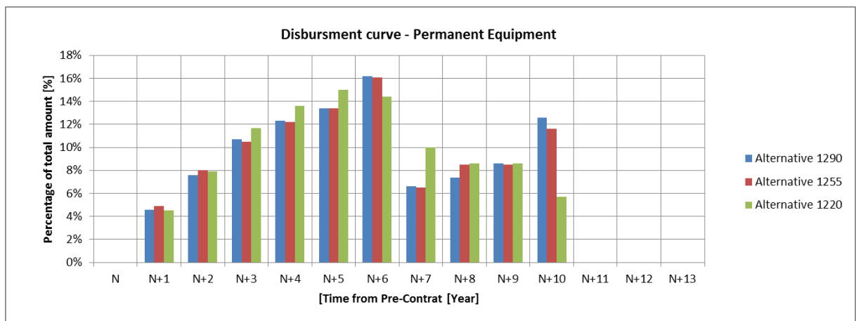
Рисунок 62: Кривая расхода – Постоянное оборудование
