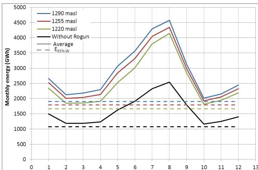
Рисунок 48 : Выработка Вахшского каскада - сравнение вариантов, сценарий (б)
