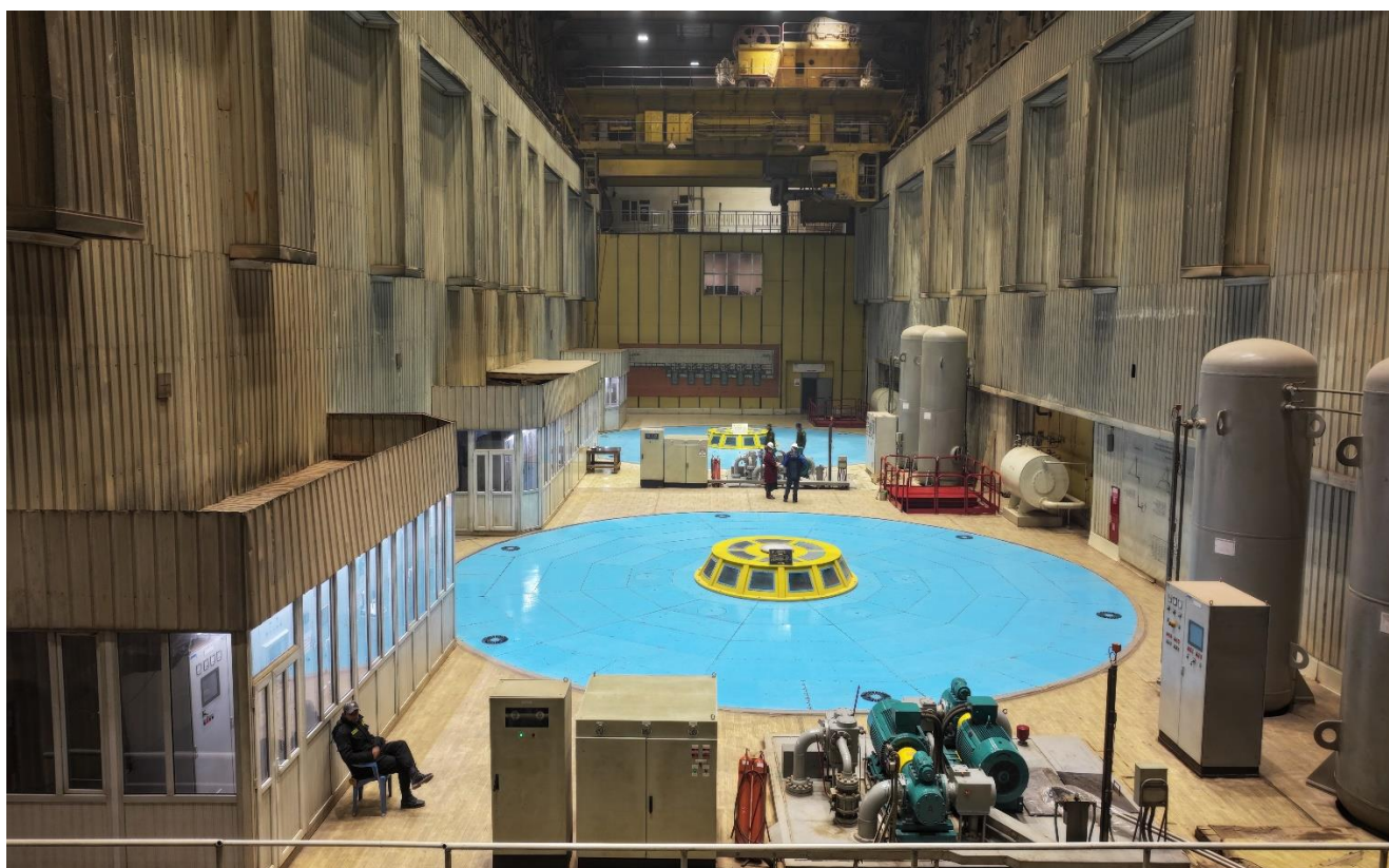
Расми 1. Ҳолати кории гидроагрегатҳои №6 ва №5.
